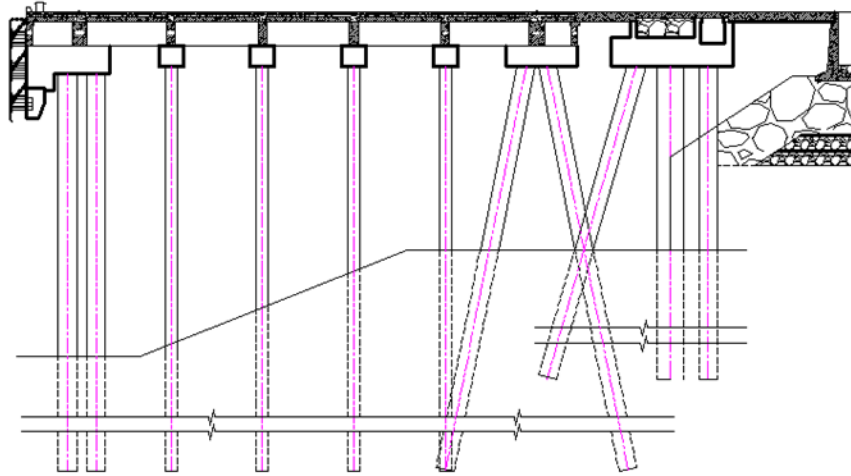
图 3.2 方案一结构形式
